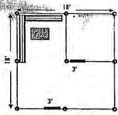
ပင်မတဲ ဆောက်လုပ်ရန် (စနစ်ပုံ)
