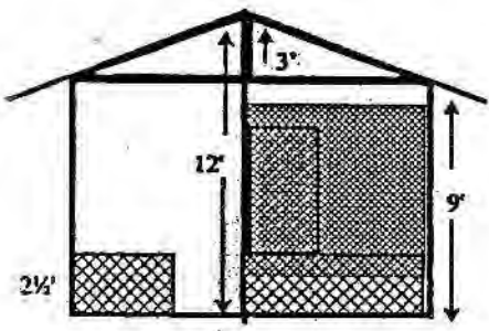
ပင်မတဲ ဆောက်လုပ်ရန်ပုံစံ (အရှေ့ဘက်မှမြင်ရပုံ)
