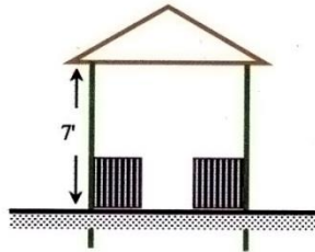
အစောင့်တဲဆောက်လုပ်ရန် (အရှေ့ဘက်မှမြင်ရပုံ)
